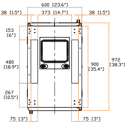
Front door
